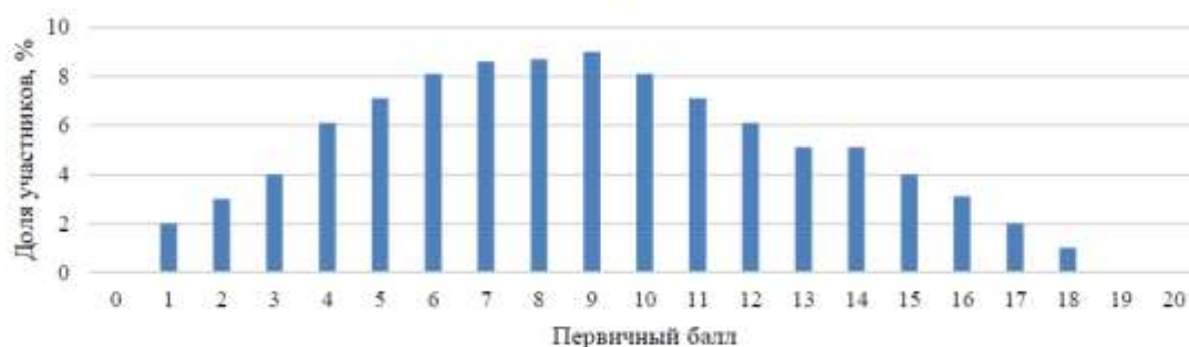
Рисунок 5. Распределение первичных баллов близкое к нормальному
